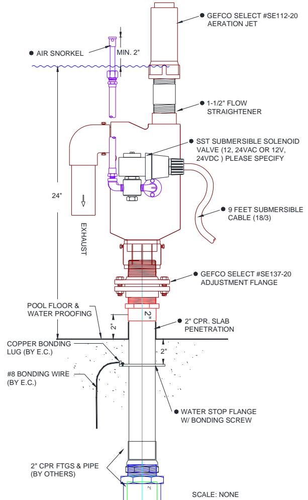
SCALE: NONE
